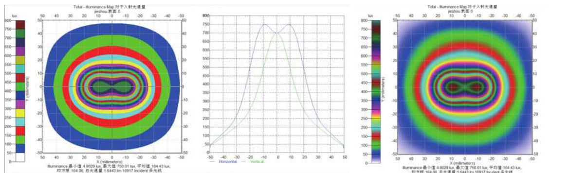
(b) 两 LED 间距 d=30mm 时光照度分布图、光照度直方图、光照度渐变图
