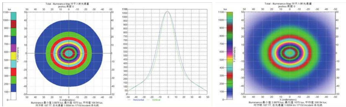
(a) 两 LED 间距 d=28mm 时光照度分布图、光照度直方图、光照度渐变图
