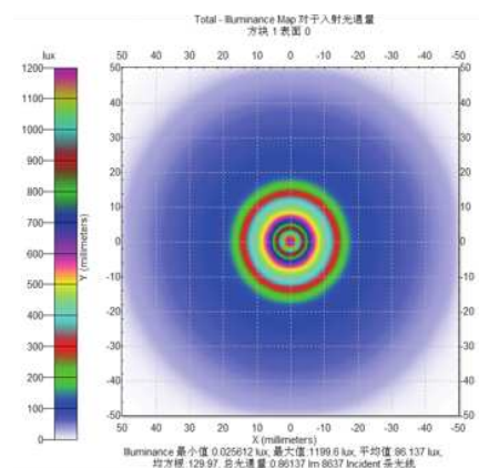
图 2 单个 LED 的光照度渐变图
