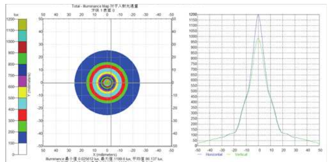
图 1 单个 LED 的光照度分布图
