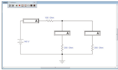
图 1 基于 DBL 教学法电路设计
