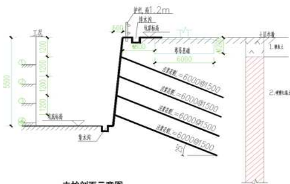
支护剖面示意图
